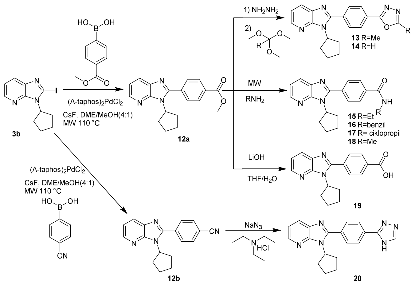
Shema 7. Sintaza ključnih spojeva 13 - 20
