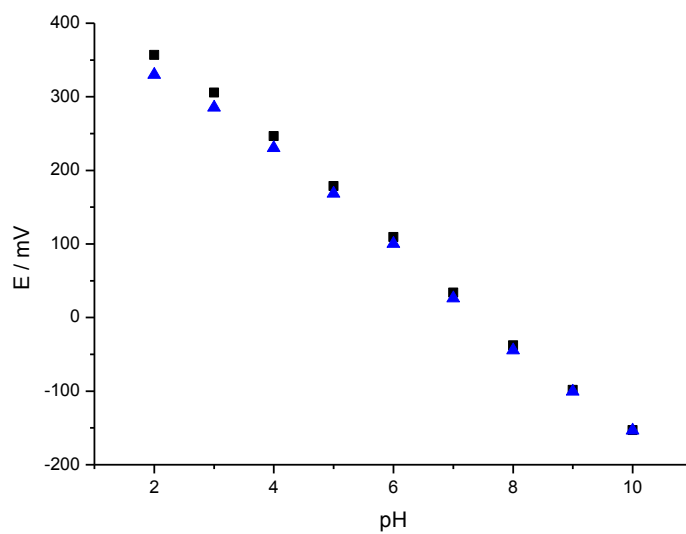
Slika 32. Baždarni dijagram za GC/polianilinsku elektrodu snimljeno 24 sata nakon pripreme senzora. Trokutići predstavljaju snimanje iz kiselog u lužnato a kvadratići iz lužnatog prema kiselo područje.
