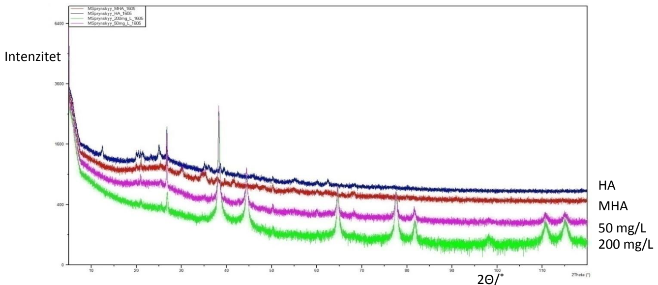
Slika 36: Uspoređba difraktograma nemođificirane huminske kiseline (HK), modificirane huminske kiseline (MHK) te sintetiziranih nanokompozita inicijalnih koncentracija c(\text{Ag}^+)=50 i 200 \text{ mg/L}
