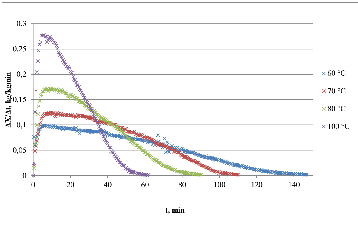
Slika 19. Grafički prikaz ovisnosti brzine sušenja uzorka celera o vremenu sušenja pri 60 °C, 70 °C, 80 °C i 100 °C
