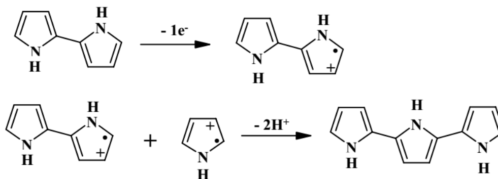
Slika10. Mehanizam oksidacije i polimerizacije polipirola
