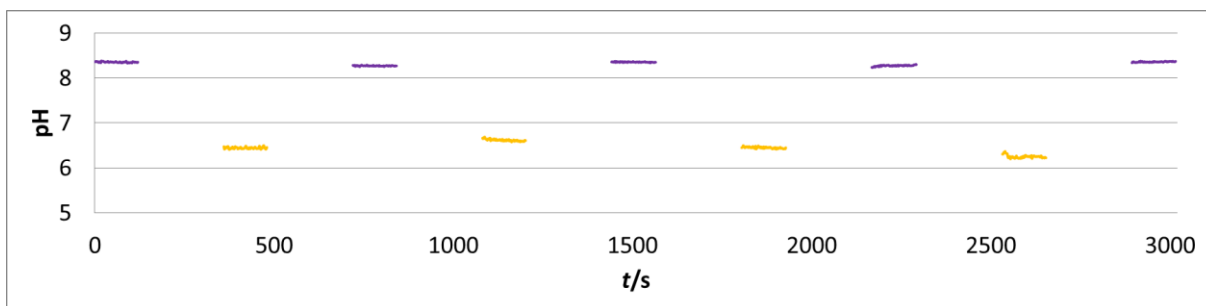
Slika 21. Dinamički odziv GJM-534 pH osjetljivog bojila imobiliziranog na zavoj uz uzastopnu promjenu pH između 6,5 i 8,5 snimanog pri valnoj duljini 546 nm.
