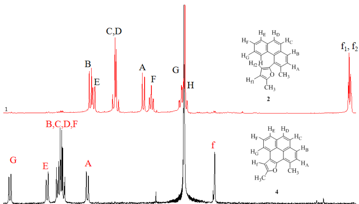
Slika 8. Usporedba ^1\text{H} NMR spektara fotoproducta 2 i 4
