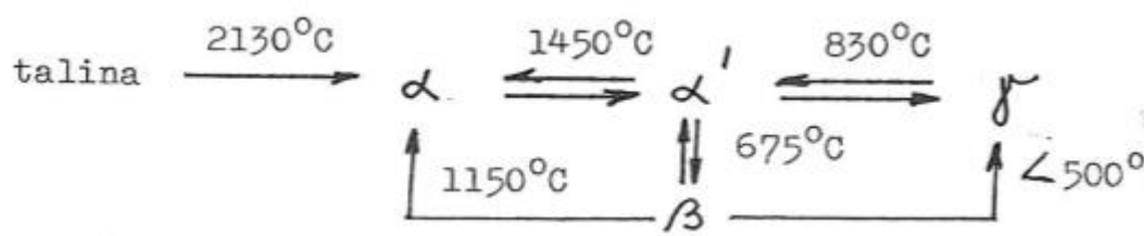
Slika 2. Polimorfne modifikacije belita
