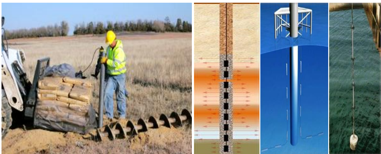
Slika 13. Duboko anodno ležište s koksnim punilom u tlu [19,20] i bez punila u moru [21]
