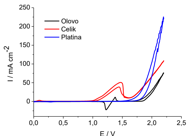
Slika 5.1. Usporedba cikličkih voltamograma dobivenih tijekom polarizacije elektroda od raznih materijala u modelnoj otopini \text{CuSO}_4
