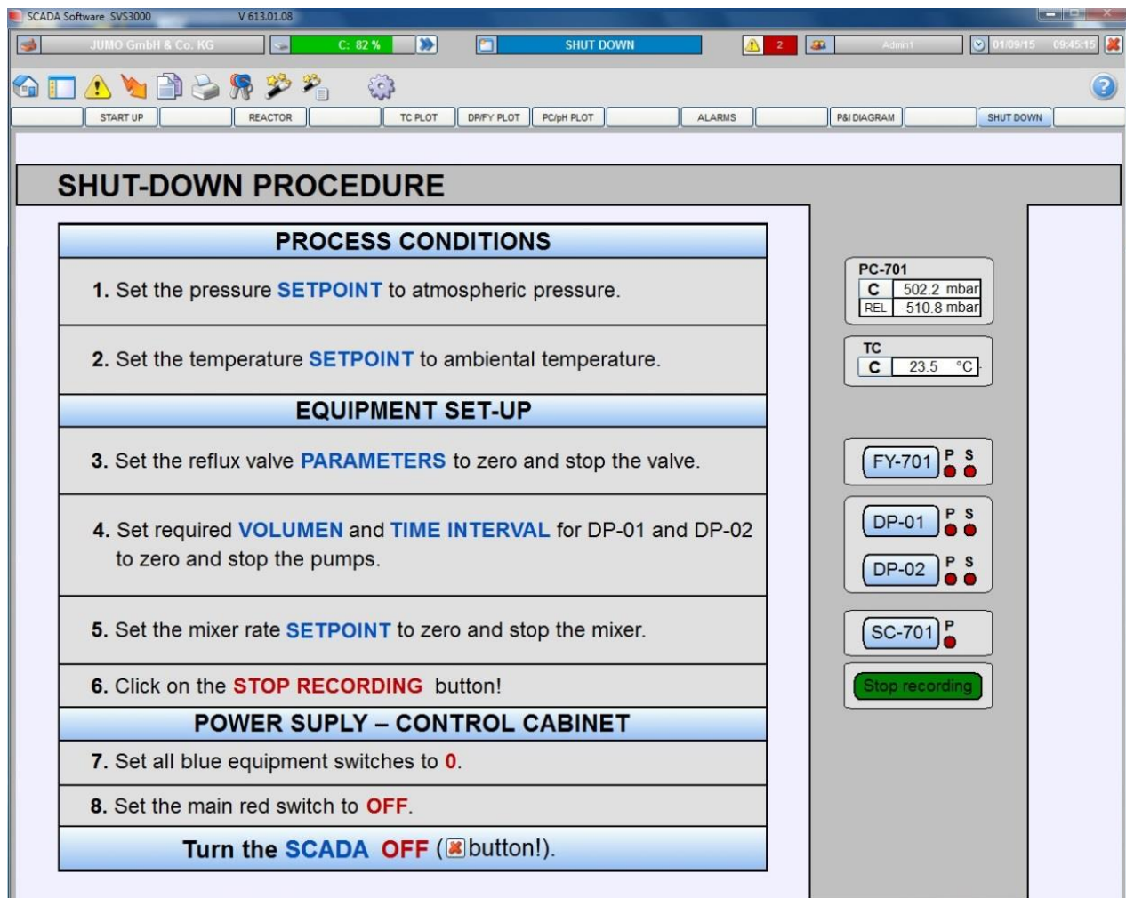
Slika 22 SHUT-DOWN sučelje
