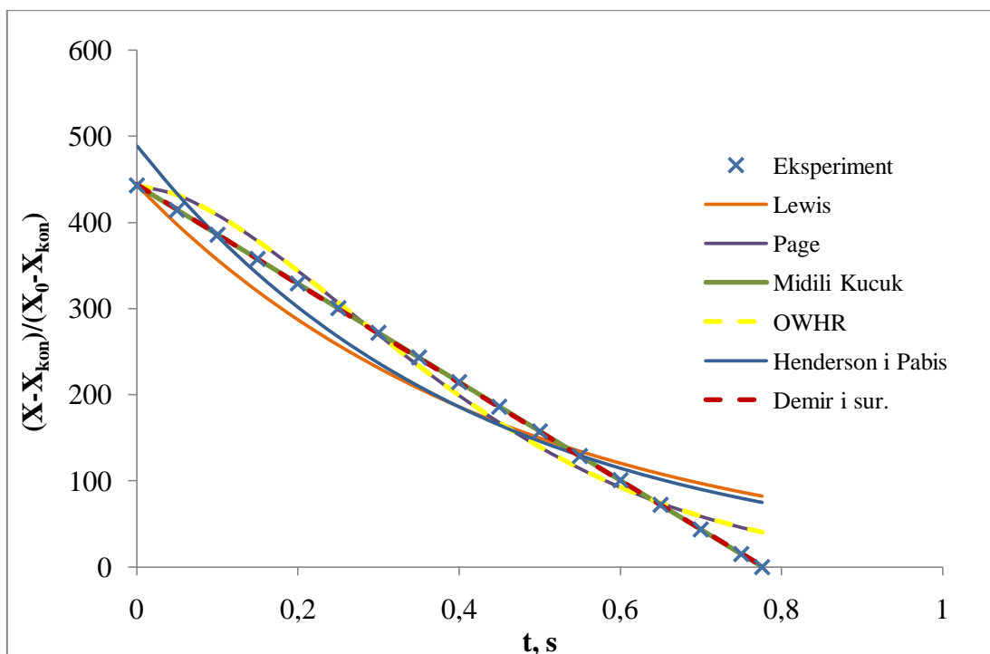
Slika 52. Aproximacija eksperimentalnih podataka sušenja uzorka iz jezera Jarun odabranim matematičkim modelima (uzorak: jarun 2)
