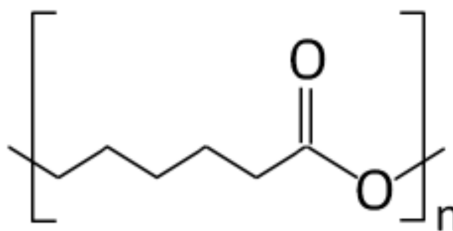
Slika 2 Struktura PCL-a[19]
