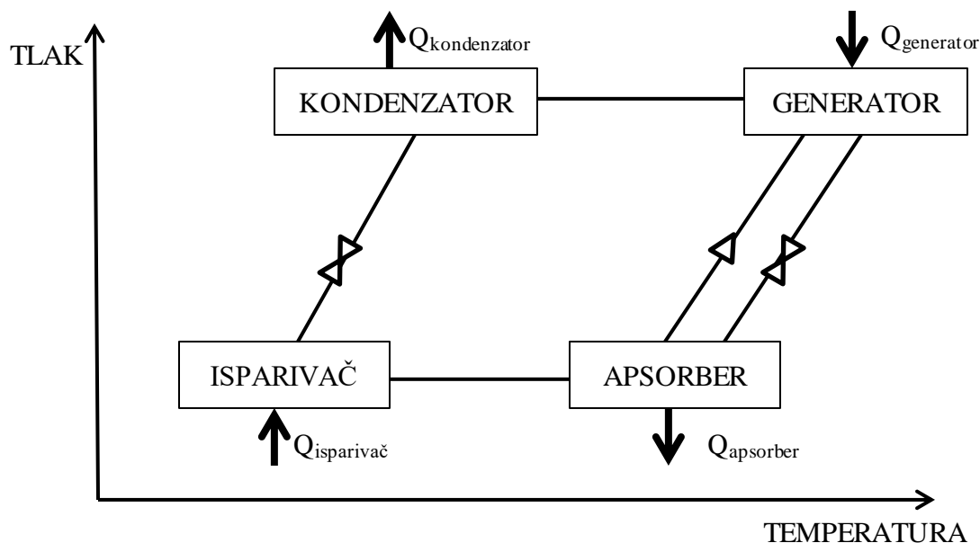
2.5. Dühringov dijagram za jednostupanjski apsorpcijski sustav [10]
