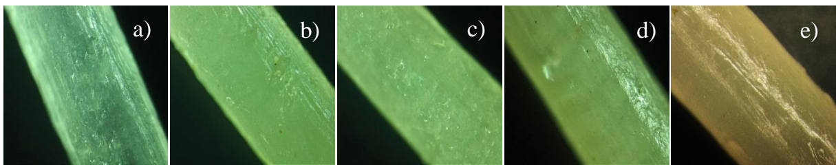
Slika 39. Mikrografija filamenata, uvećanje 64x: a) F5%, b) F10%, c) F15%, d) F20% i e) F10%P
