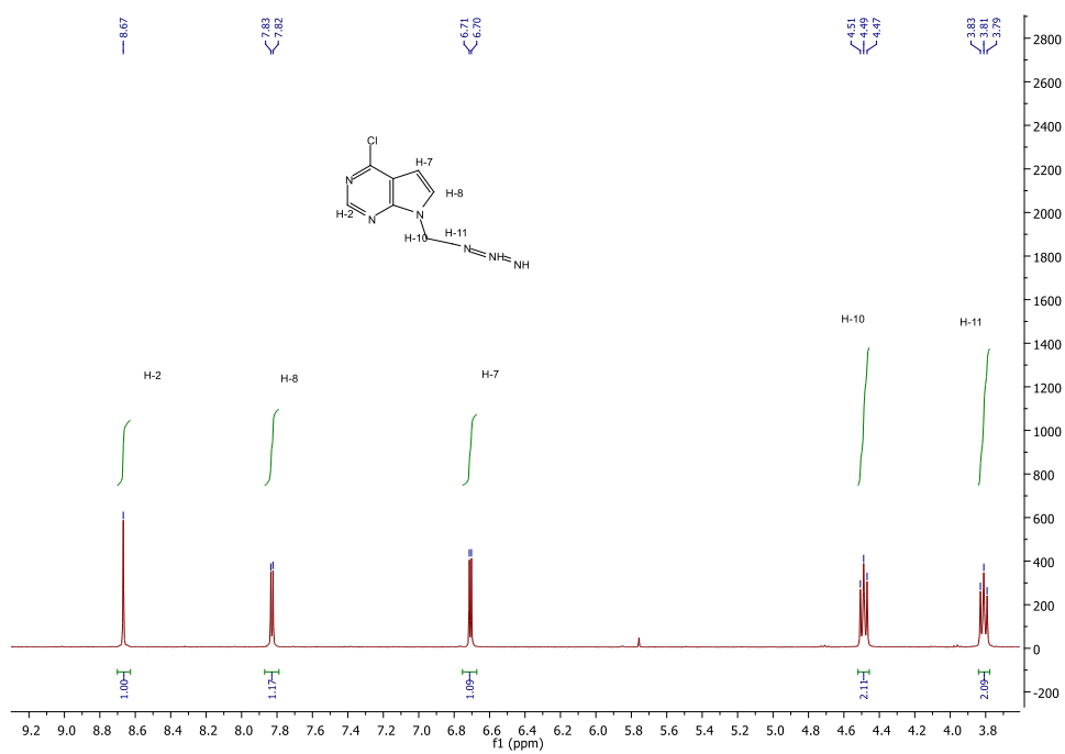
Slika 21. ^1\text{H} NMR spektar spoja 2
