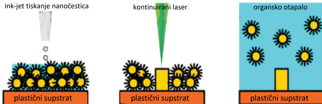
Slika 4. Selekтивно lasersko sinteriranje NP-a ink-jet tiskanih na polimernoj podlozi. 4
