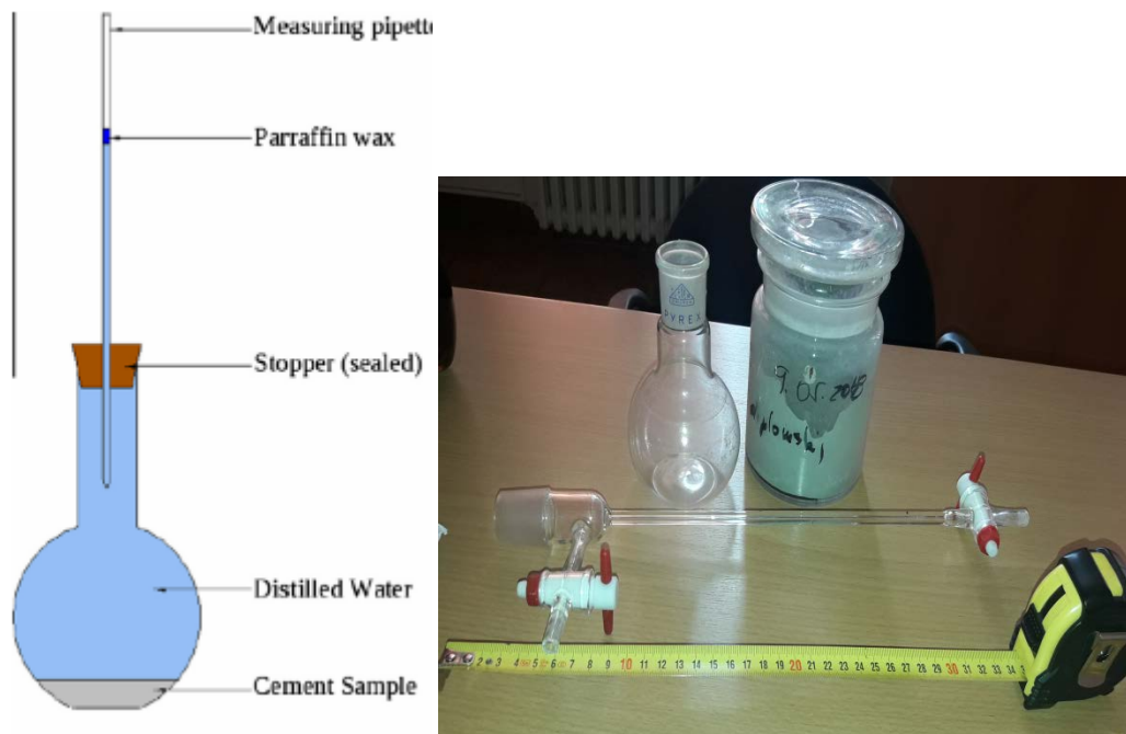
Slika 13. Shematski prikaz piknometrijskog mjerenja kemijskog skupljanja (lijevo), te dijelovi aparature s ubrušenim čepom i teflonskim pipcima za lakše odzračivanje.
