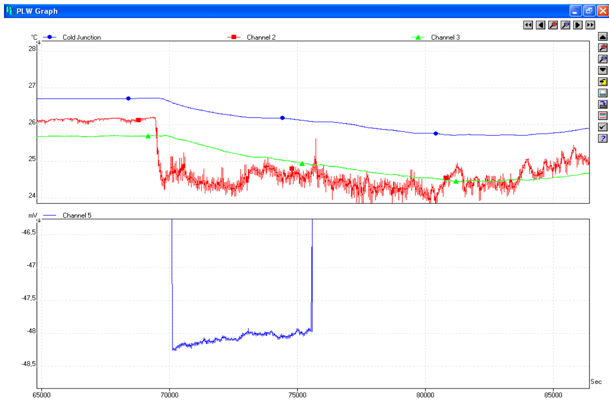
Slika 27. Detalj mjerenja od 70000 do 75500 s, pri konstantnoj masi, no uz promjenu temperature parafina veću od oko 0.7 °C.
