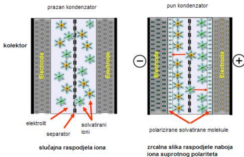
Slika 2.7. Shema procesa punjenja i pražnjenja superkondenzatora
