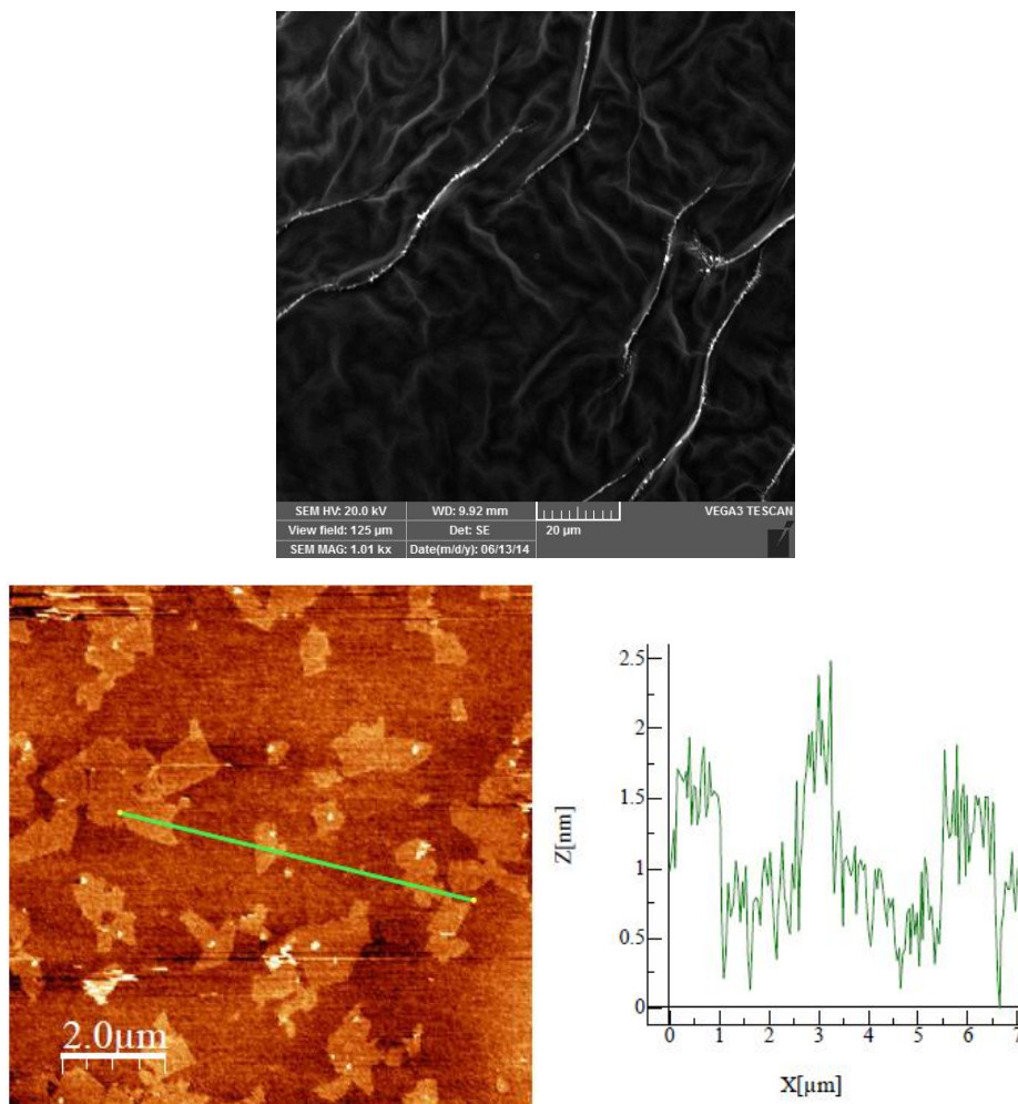
Slika 3.1. a) SEM snimka uzorka GO i b) AFM snimka uzorka GO.
