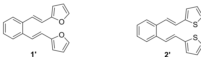
Slika 1. Difuranski i ditiofenski derivati stilbena.
