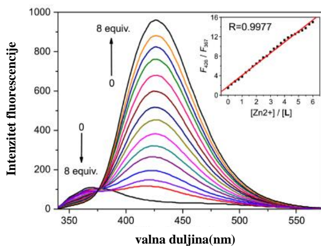
Slika 10. a) Promjene u emisijskom spektru spoja L dodatkom različitih metalnih kationa; b) Povećanje intenziteta fluorescencije postupnim dodatkom Zn^{2+} iona u otopinu spoja L. [8]
