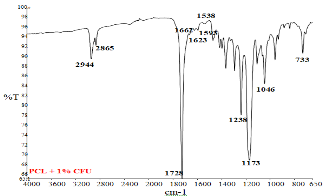
Slika 19. FTIR spektar PCL + 1% CFU vlaknastog nosača
