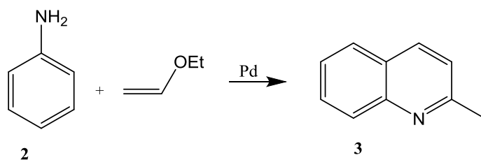
Shema 6. Sinteza spoja 3
