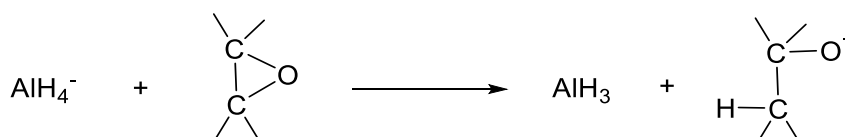
Shema 10. Mehanizam reakcije otvaranja epoksida hidridom.
