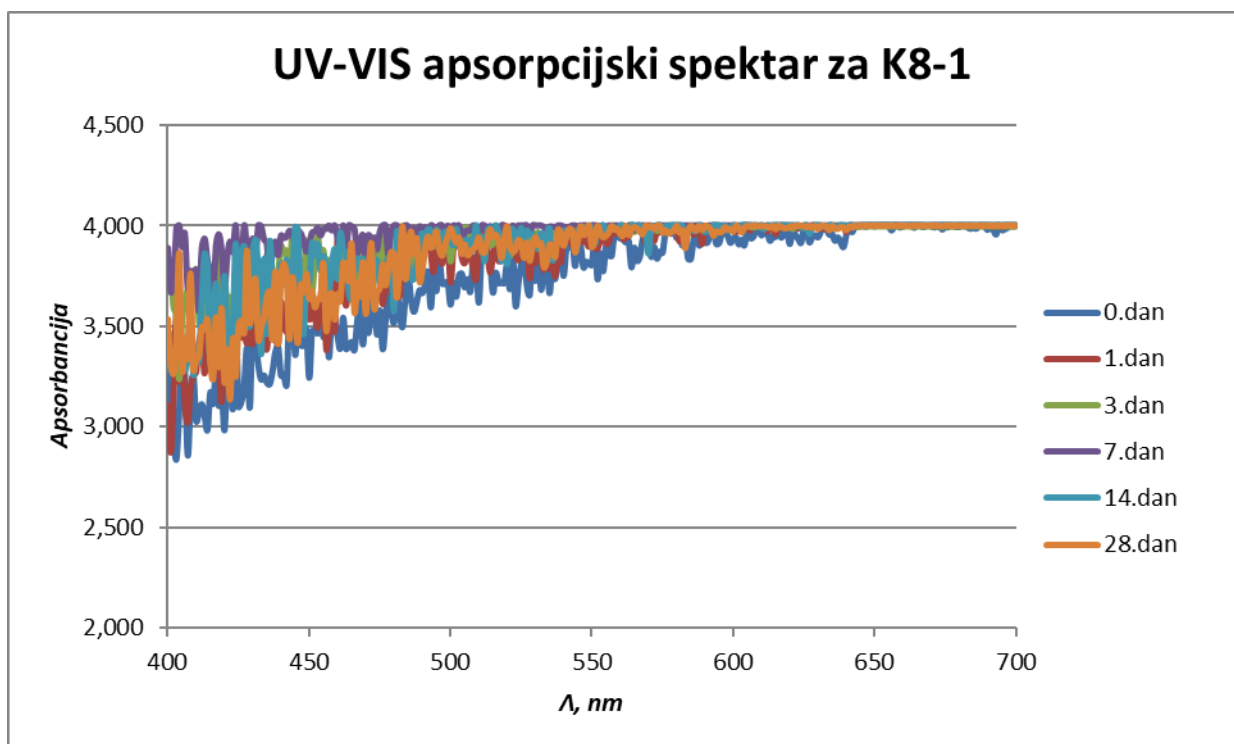
Slika 3.2.9. UV-VIS apsorpcijski spektar za uzorak K8-1
