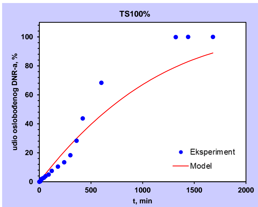
Slika 52. Oslobođanje DNR-a iz tablete TS100% – usporedba eksperimentalnih vrijednosti i Hixson – Crowellova modela
