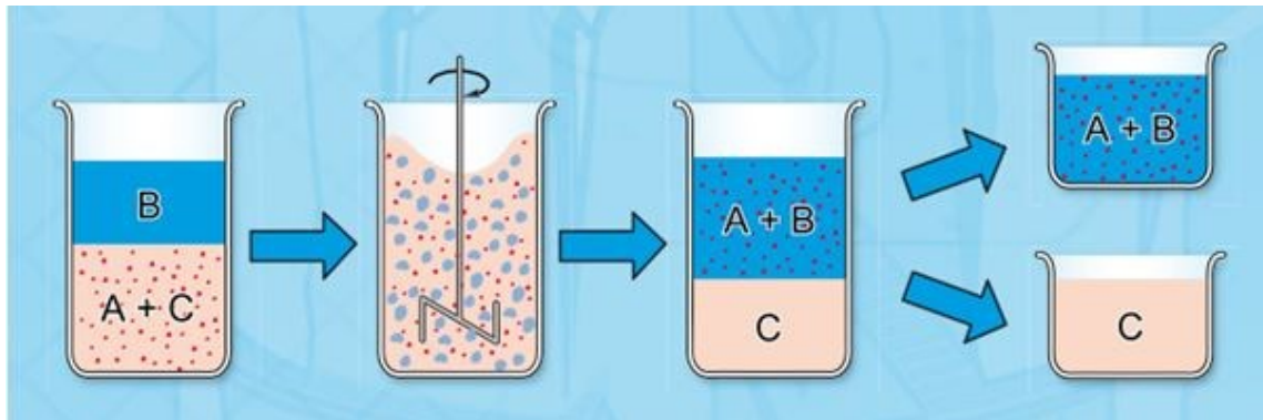
Slika 9. Shema procesa ekstrakcije kapljevitost-kapljevitost [21]
