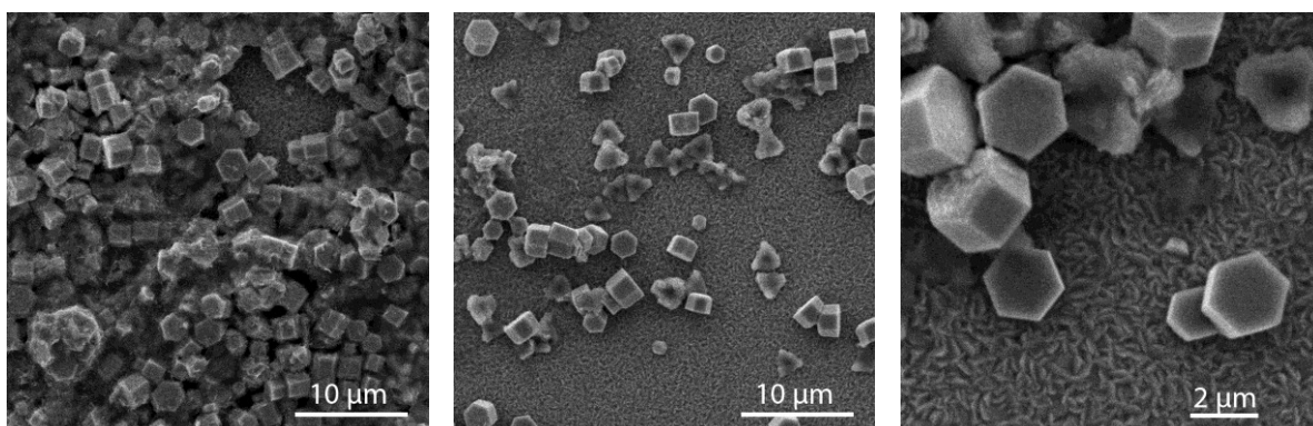
Slika 9. Prevlake dobivene iz otopine samog \text{ZnAc} \cdot 2\text{H}_2\text{O} nakon 4 h sinteze na 90 °C na podlogama sa slojem kristalnog sjemena
