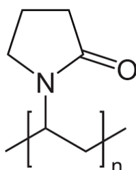
Slika 10. Strukturni prikaz poli(vinil-pirolidona)
