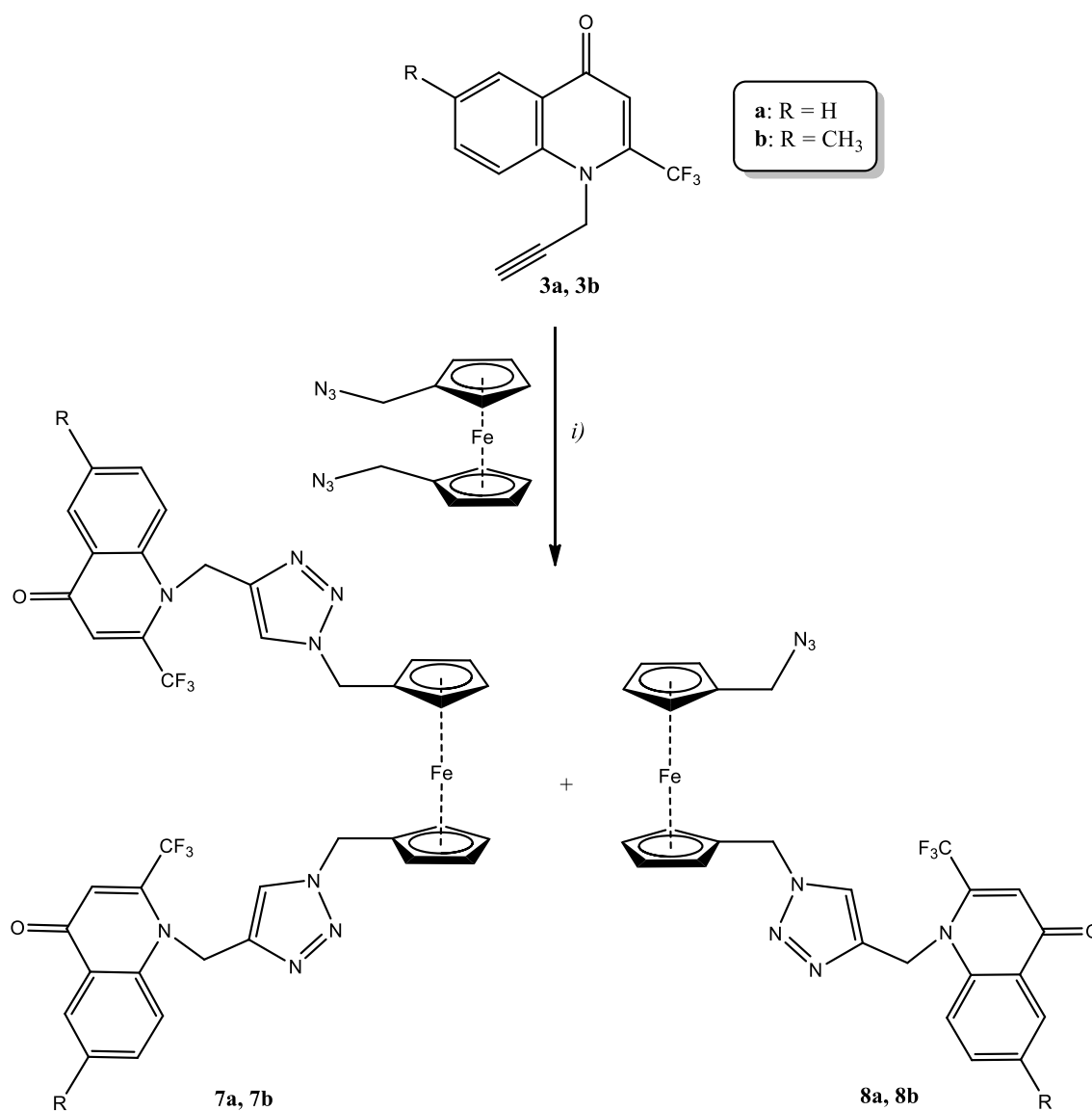
Shema 5. Reagensi i uvjeti: i) Cu(OAc) 2 , 30 μL CH 3 OH, čelična posudica, dvije čelične kuglice (promjera 7 mm), 25 Hz, 45 min.
