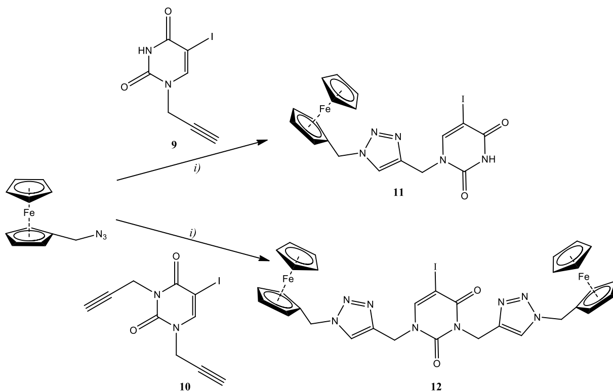
Shema 7. Reagensi i uvjeti: i) \text{CH}_3\text{OH} , \text{Cu}(\text{OAc})_2 , s.t., 24h
