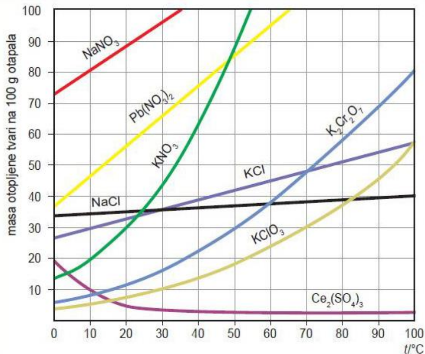
Slika 2.2. Promjena toplјivosti s temperaturom različitih tvari u vodi (krivulje toplјivosti)
