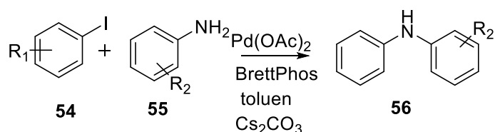
Shema 18. \text{ArI} kao nukleofil u Buchwald-Hartwigovoj reakciji.
