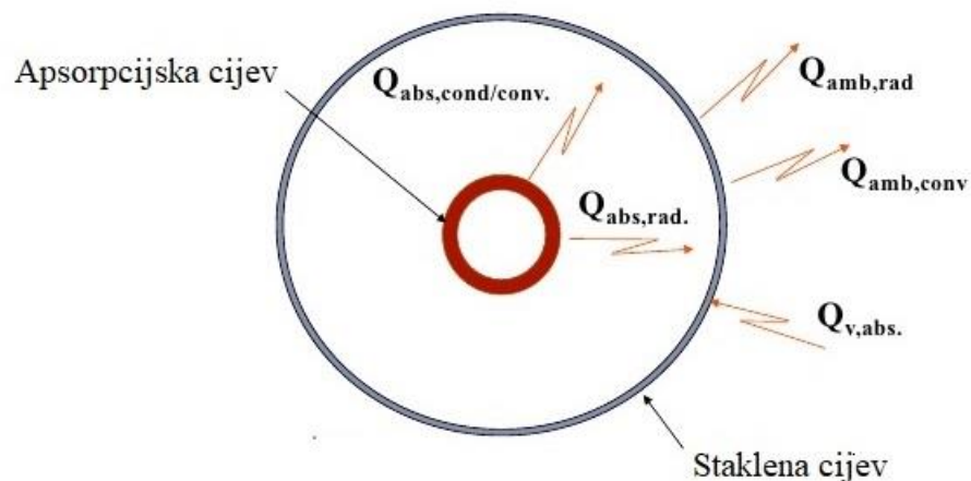
Slika 21. Energetske tokove apsorpcijske cijevi [23].
