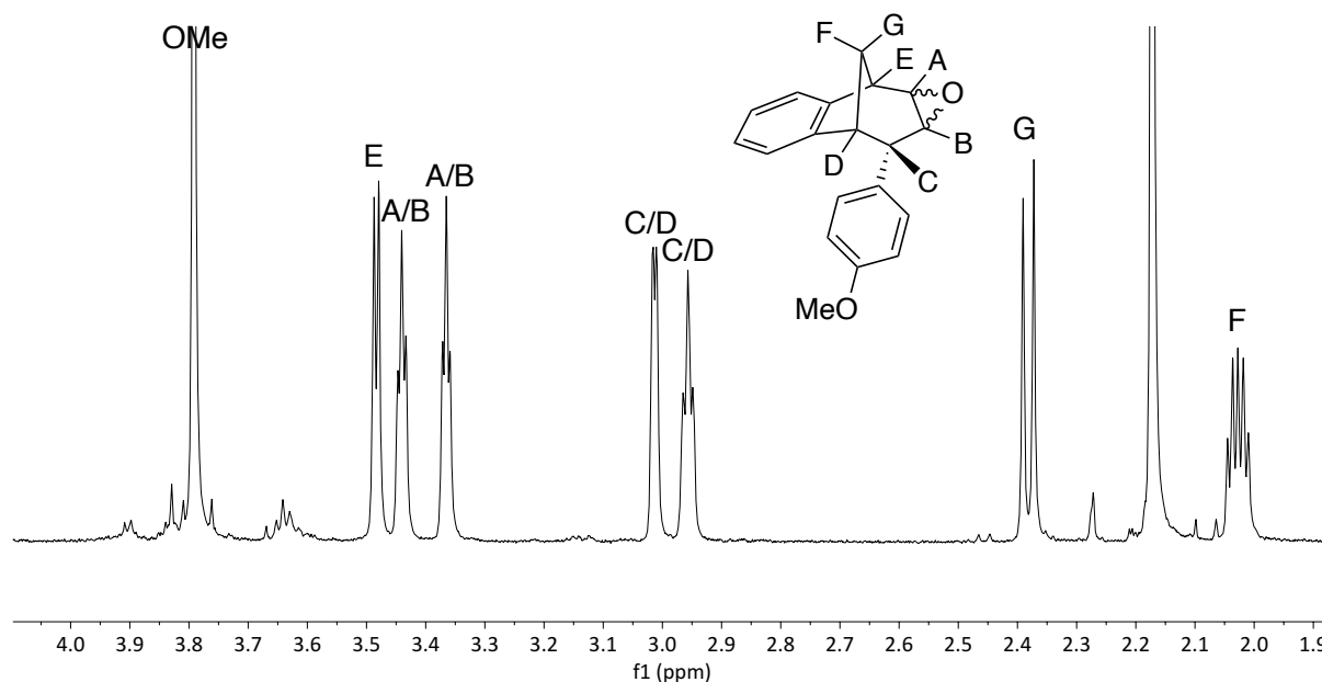
SLIKA 3.5 Dio ^1\text{H} NMR spektra epoksida 3b
