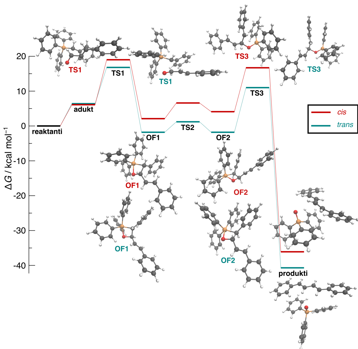
SLIKA 7.1 Energijski profil Wittigove reakcije trifenilfosfonijevog benzilida s cimnanim aldehidom
