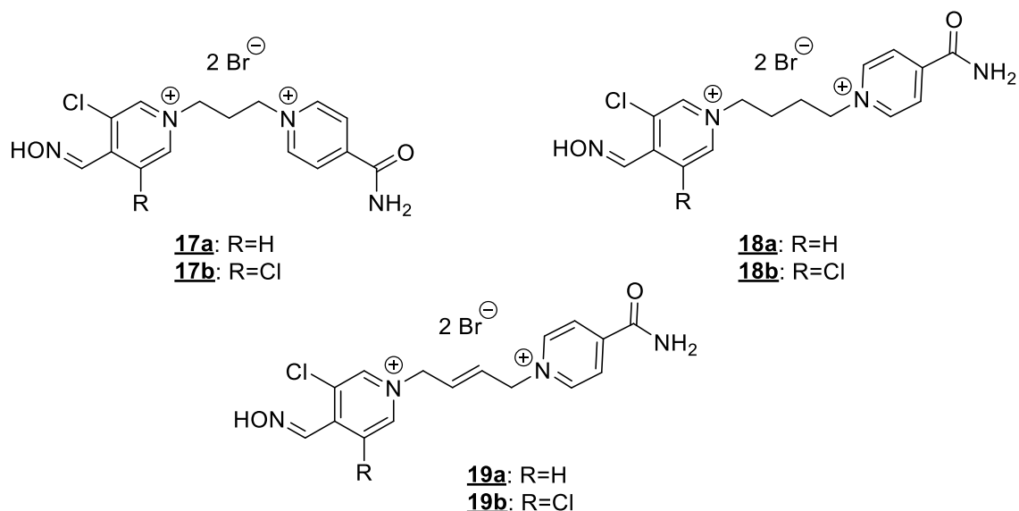
Slika 2.8. Strukture spojeva 17 – 19 .
