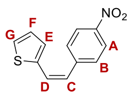
cis-5
