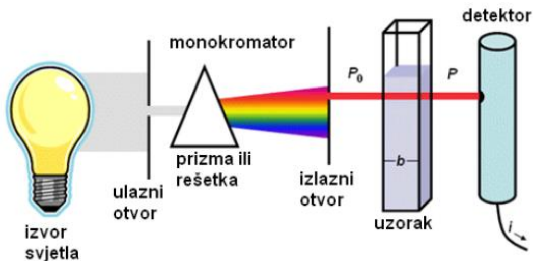
Slika 8. Shematski prikaz spektrofotometra.
