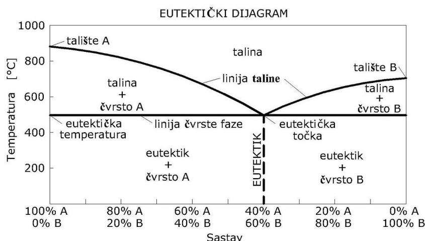
Slika 7. Eutektički dijagram.
