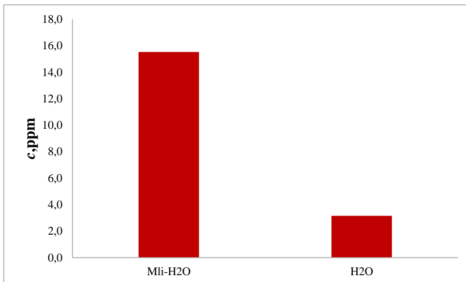
Slika 30. Rezultati ekstrakcija sa vodom i s otopinom vode i mliječne kiseline.
