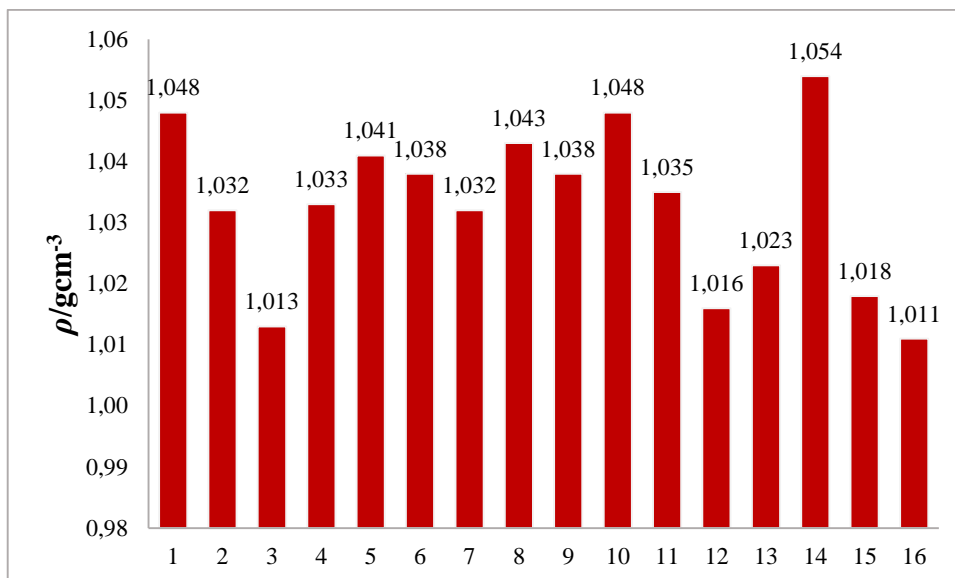
Slika 31. Usporedba vrijednosti gustoće za različite smjese otapala, \rho , gcm -3 .
