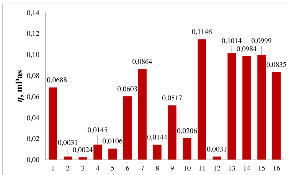
Slika 32. Vrijednosti viskoznosti za ispitane smjese otapala.
