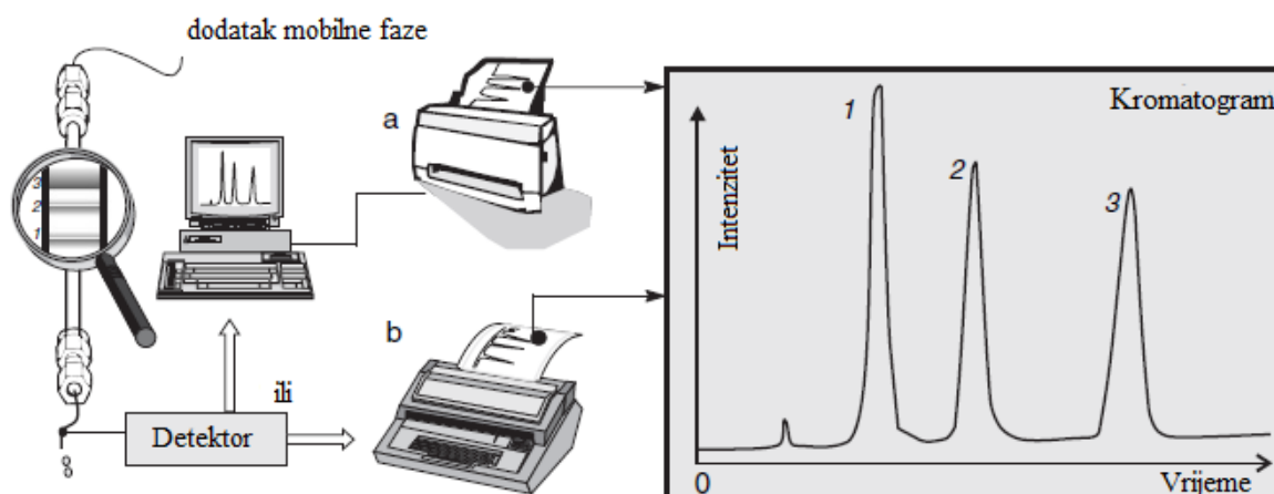
Slika 9. Shema principa analize kromatografom.
