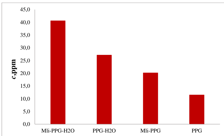
Slika 29. Prikaz rezultata ekstrakcije s različitim otapalima.
