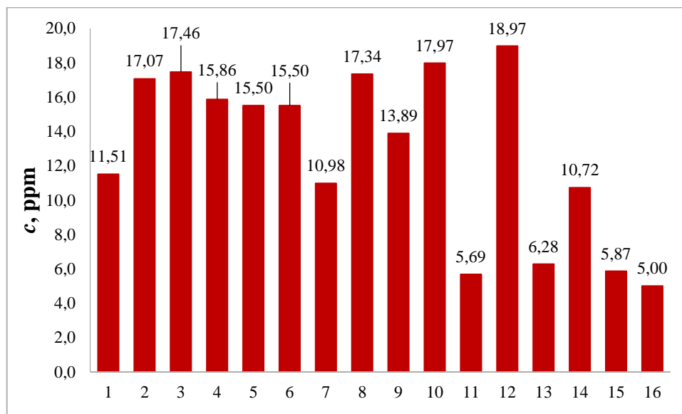
Slika 34. Koncentracija ukupnih polifenola.
