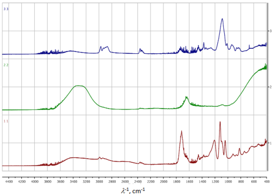
Slika 28. FTIR spektar za otapala: mliječna kiselina, —, PPG 400, — i Mli:PPG-1:2 —.
