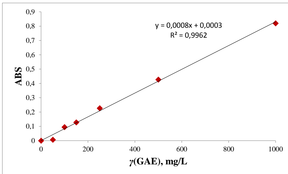
Slika 23. Baždarni dijagram galne kiseline.
