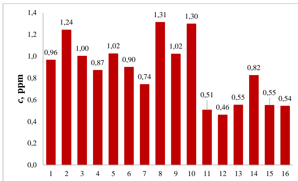
Slika 35. Grafički prikaz koncentracije oleuropeina u ekstraktima.
