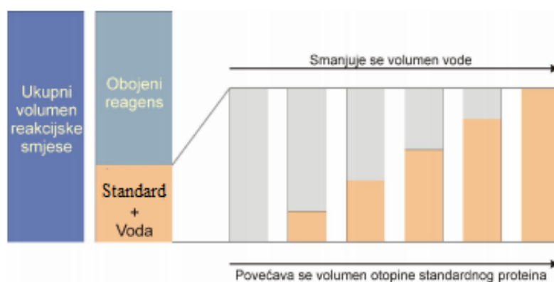
Slika 22. Shematski prikaz određivanja baždarnog dijagrama za određivanje koncentracije ukupnih polifenola.
