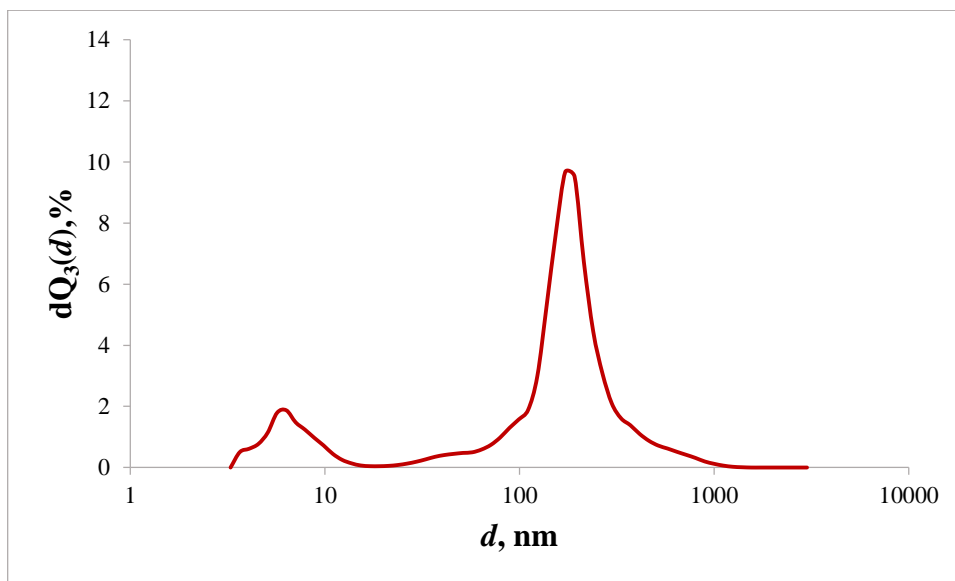
Slika 27. Raspodjela veličina čestica lišća.
