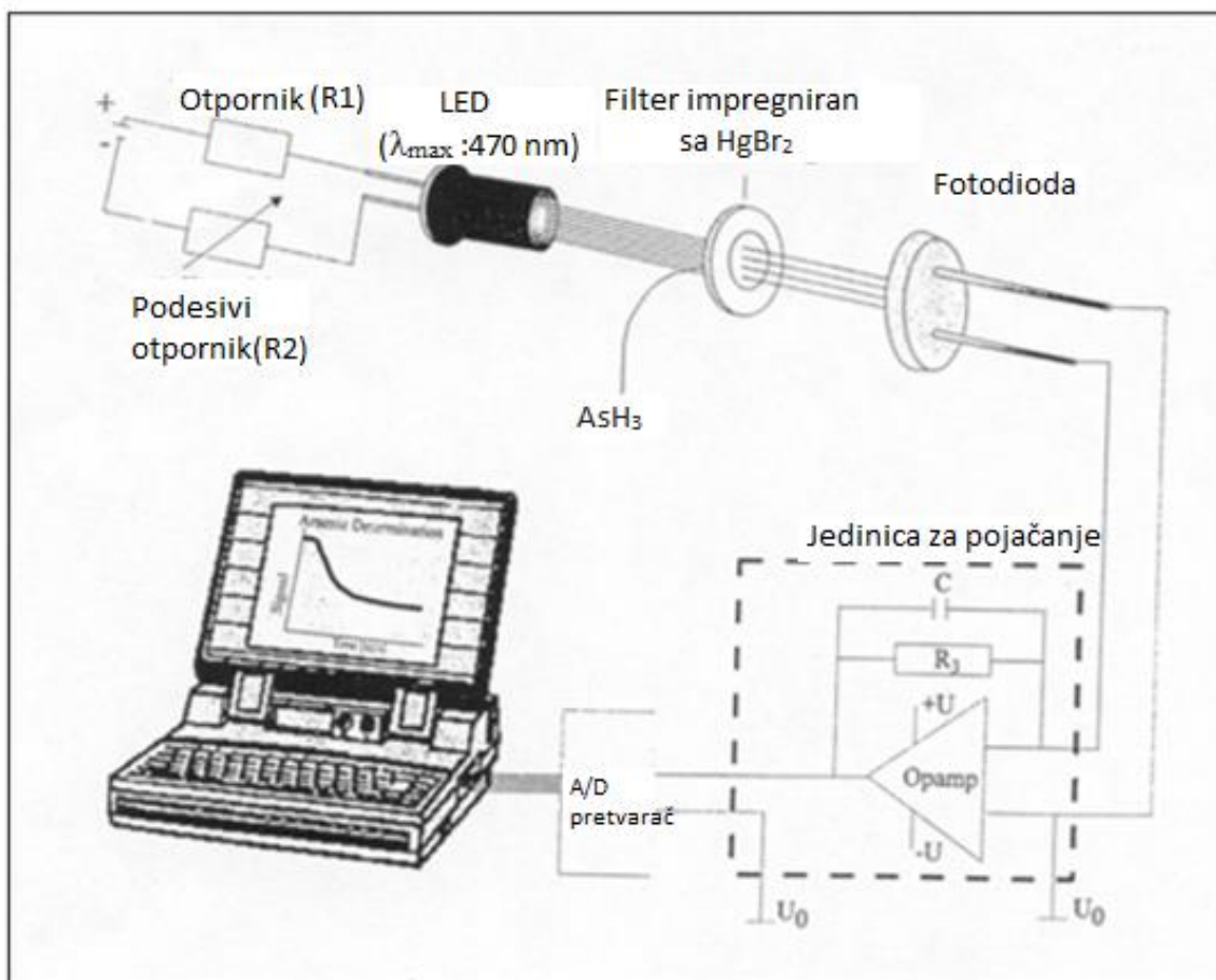
Slika 3.: Shema uređaja [14]
