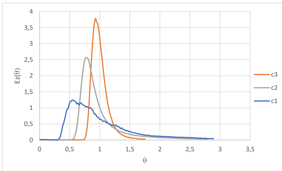
Slika 4.7. Promjena cijevi uz konstantan protok od 136 ml/min
