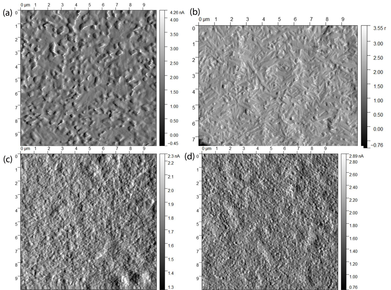
Slika 72. AFM mikrografije (a) FAPI perovskita bez PVP-a i (b) FAPI perovskita sa 8 \text{mg ml}^{-1} PVP-a aniliranog pri 200 ^{\circ}\text{C} te (c) \text{Cs}_{0.1}\text{FA}_{0.9}\text{PbI}_3 perovskita bez PVP-a i (d) \text{Cs}_{0.1}\text{FA}_{0.9}\text{PbI}_3 perovskita sa 8 \text{mg mL}^{-1} PVP-a aniliranog pri 150 ^{\circ}\text{C} .
