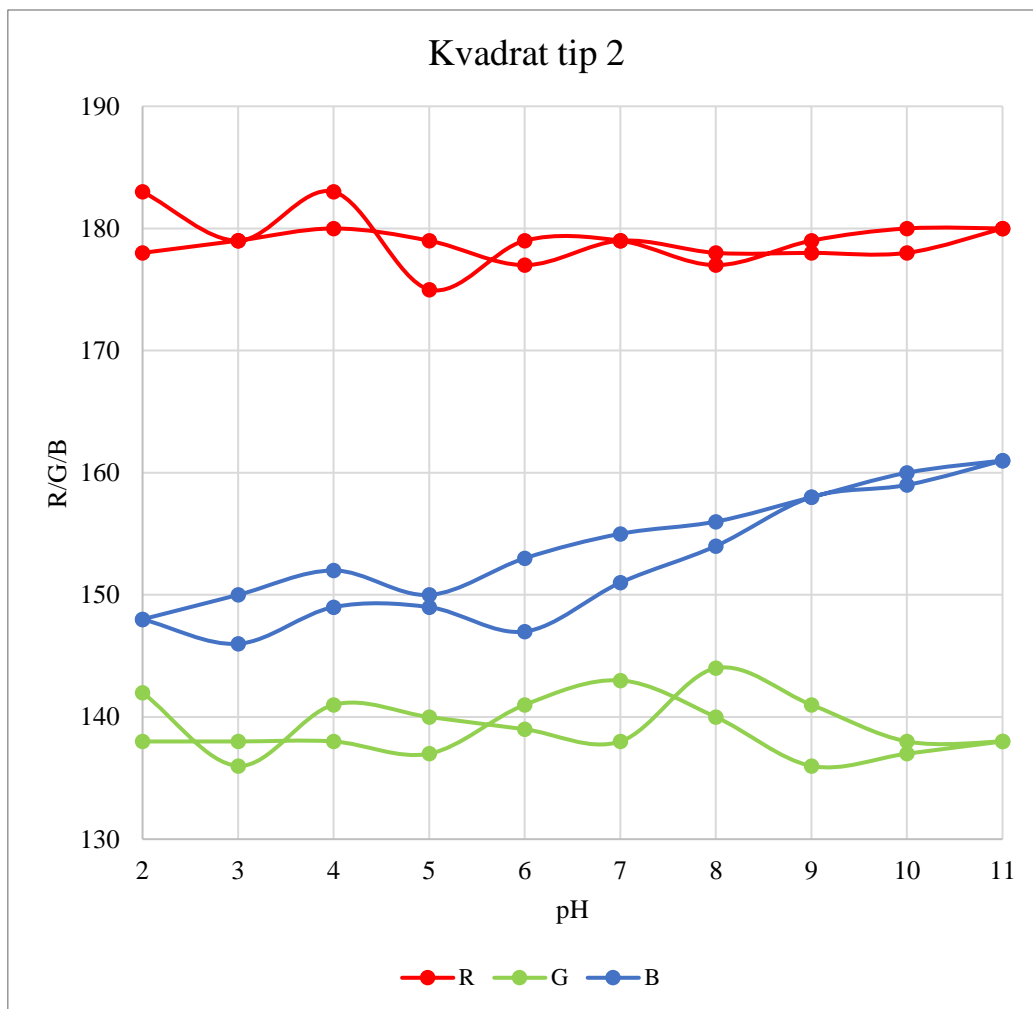
Slika 62. RGB vrijednosti za mikroreaktor tipa 2 s kvadratnim presjekom kanala
