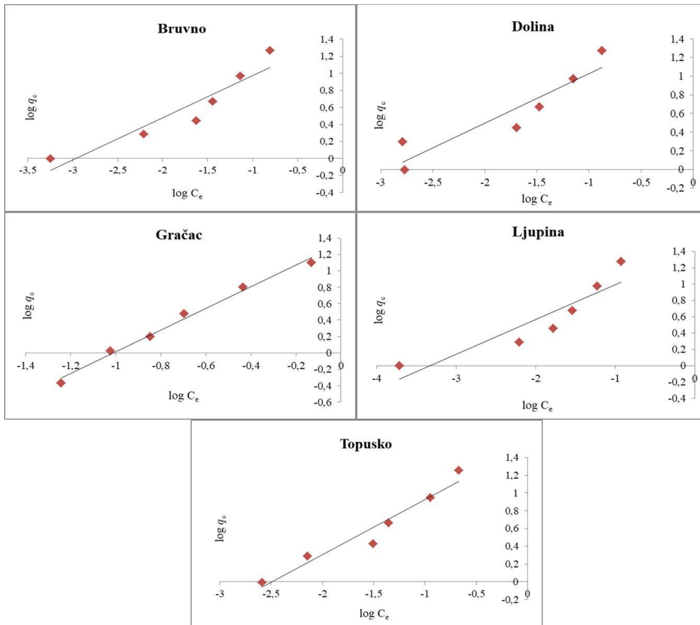
Slika 4.5. Prikaz Freundlichovih sorpcijskih izoterma trimetoprma na uzorcima tla
