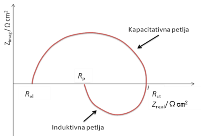
Slika 2.6.8. Nyquistov dijagram za jednostavan elektrokemijski sustav.
