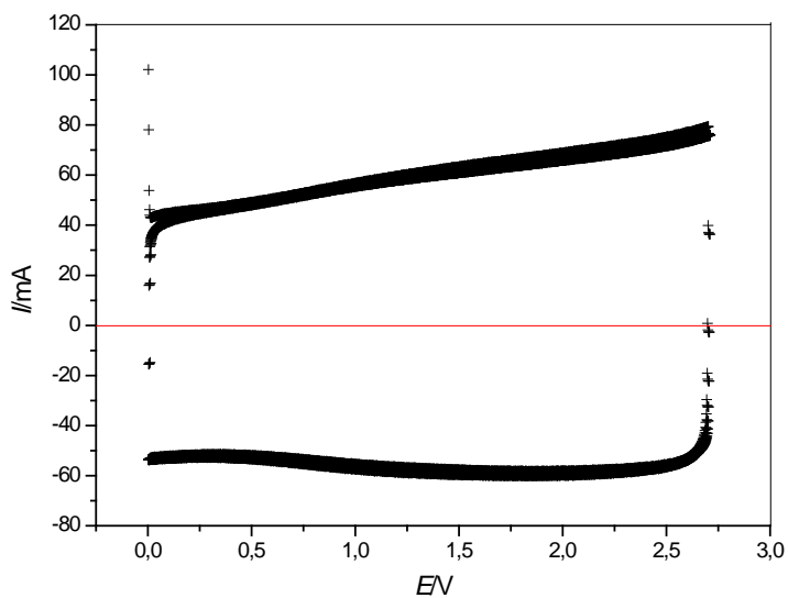
Slika 4.11. Ciklički voltamogram za superkondenzator nominalnog napona od 2,7 V.
