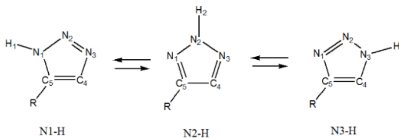
Slika 11. Tautomeri 1,2,3-triazola
