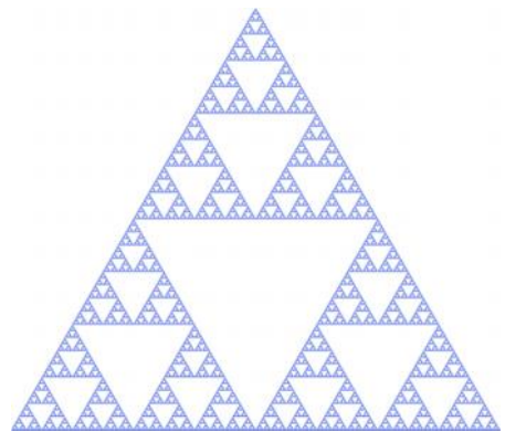
Slika 3.9. Trokut Sierpinskog
