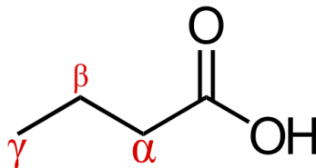
Slika 1. Prikaz \alpha i \beta ugljika u organskoj molekuli. 10
