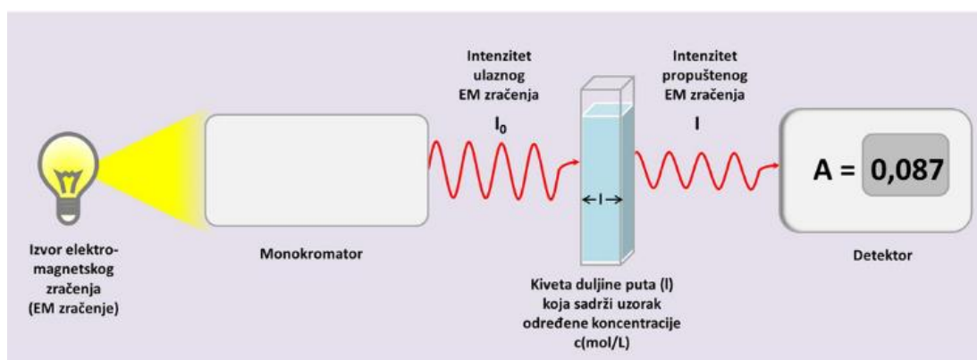
Slika 9. Princip mjerenja apsorbcije na UV/VIS spektrofotometru [12]
