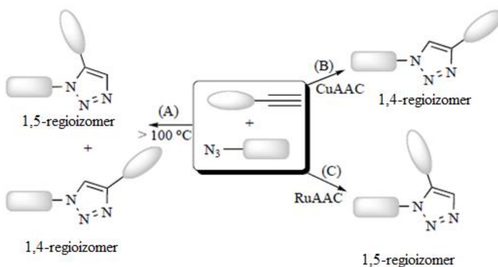
Shema 4. Bakrom (CuAAC) i rutenijem (RuAAC) katalizirane Huisgenove cikloadicije
