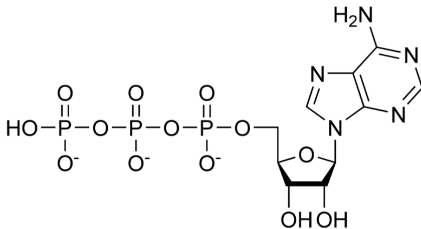
Slika 4. Struktura ATP-a
