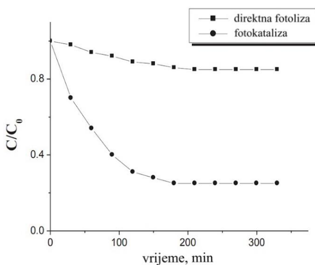
Slika 11. Usporedba raspada onečišćujuće tvari direktnom fotolizom i \text{TiO}_2/\text{UV} metodom. [24]
