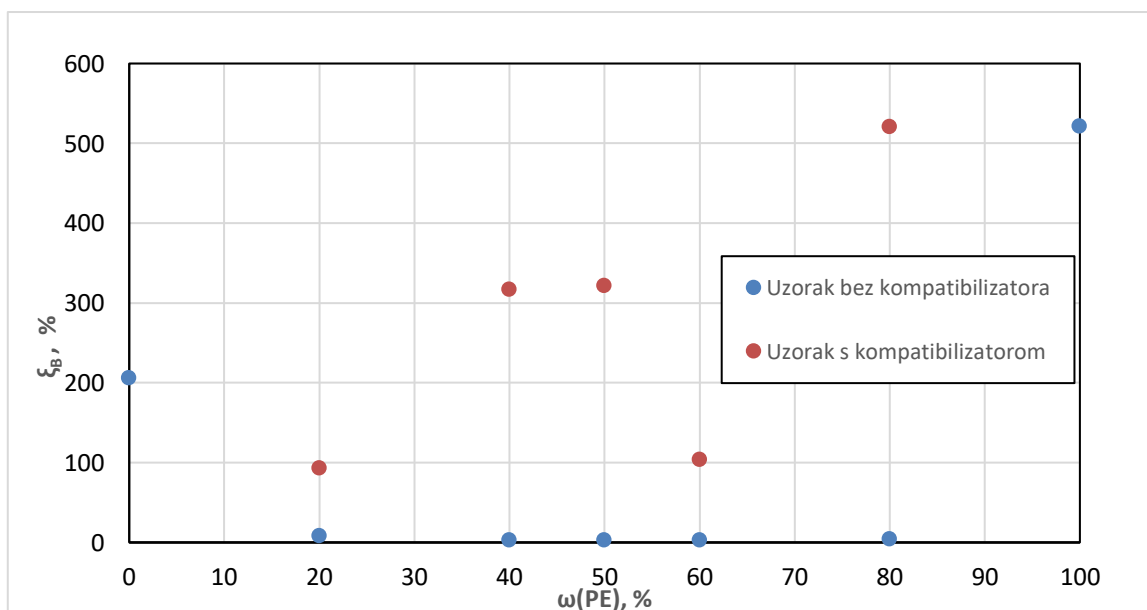
Slika 25. Ovisnost prekidnog istežanja o masenom udjelu polietilena u uzorcima
