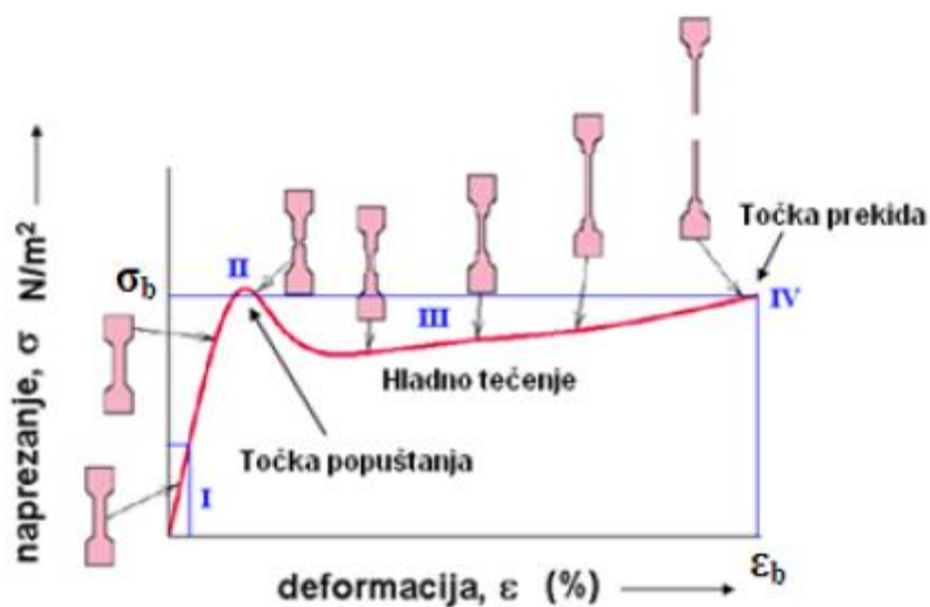
Slika 1. Dijagram napreznje-istezanje[6]
