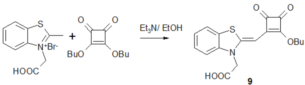
Slika 27. Sinteza spoja 9 [23].
